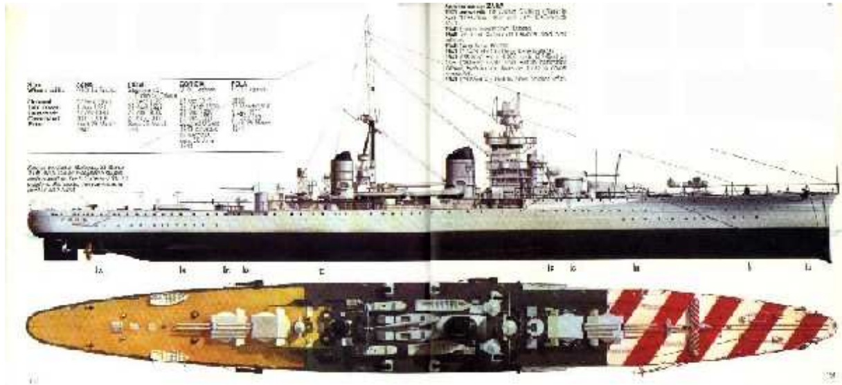
Profilo longitudinale pianta dell'unità
